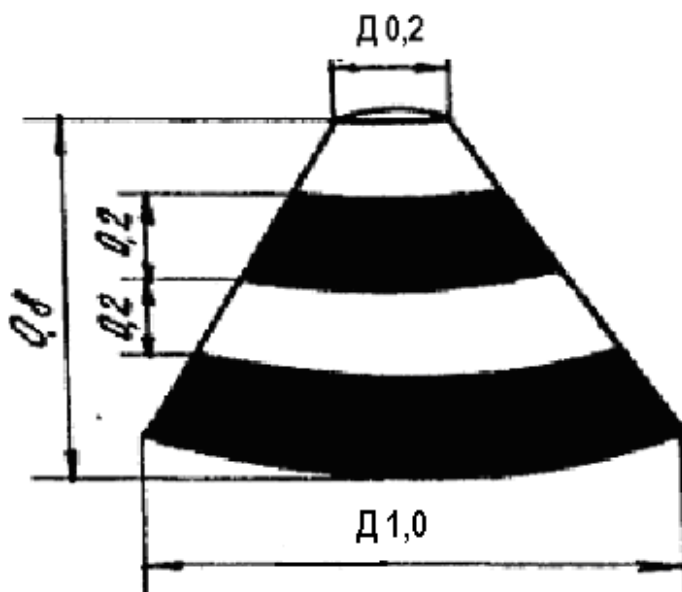
Рис. П.4.4 Пограничный маркер
