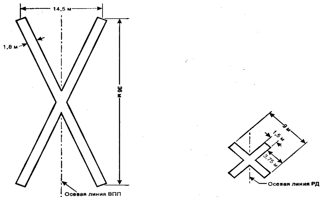
Рис. 5.7. Маркировка закрытых для движения ВПП и РД.
