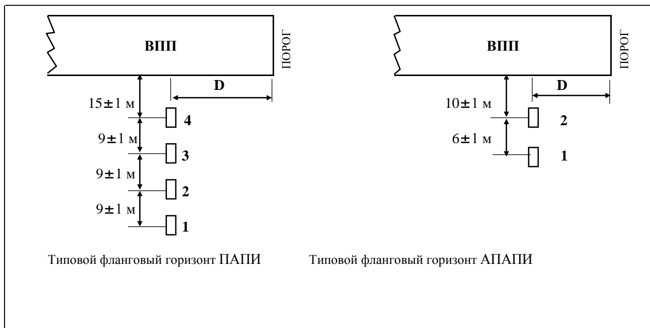
Рис. 5.22. Расположение систем ПАПИ и АПАПИ
