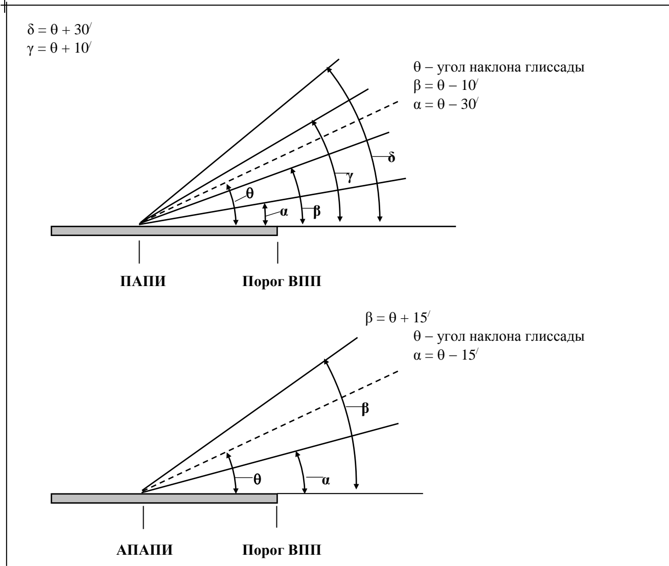
Рис. 5.23. Углы возвышения огней в системах ПАПИ и АПАПИ (для углов наклона глиссады 2^\circ - 4^\circ )
