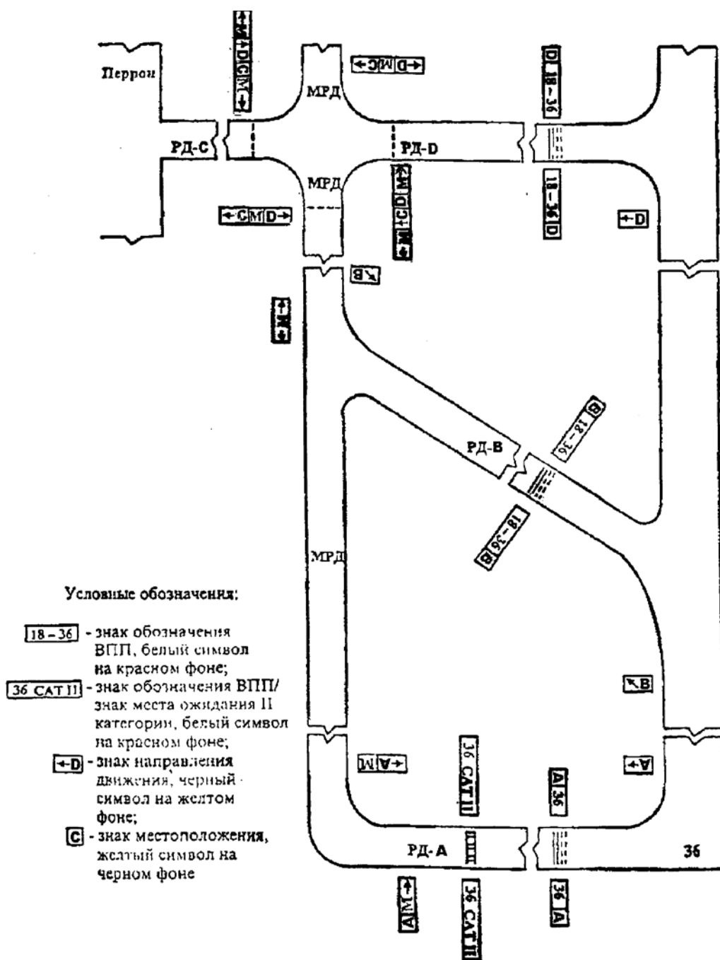
Рис. П.6.4. Пример расположения аэродромных знаков.
